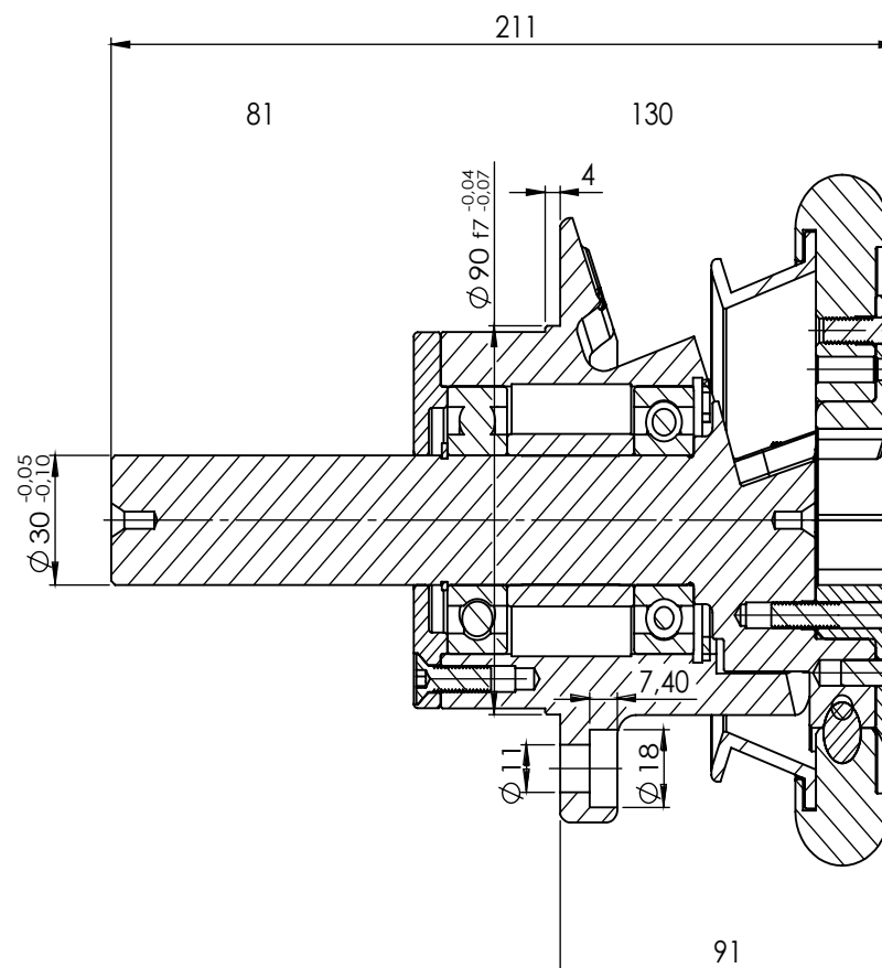
SECTION A-A SCALE 2:3
